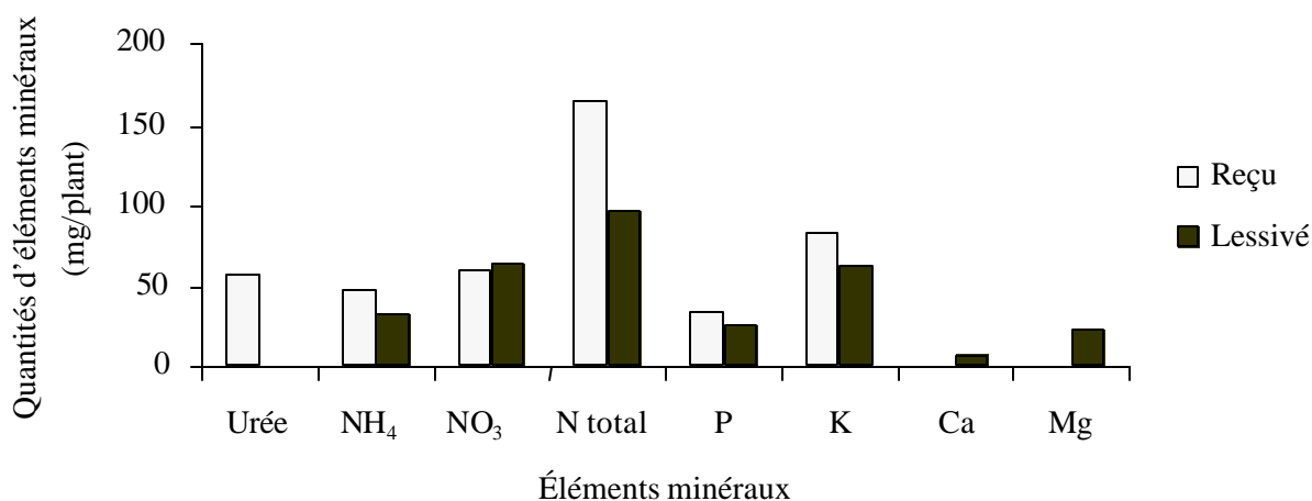
Figure 3. Quantités d'éléments minéraux (mg/plant) reçues et lessivées sous la culture extérieure d'épinette blanche 2 + 0.
