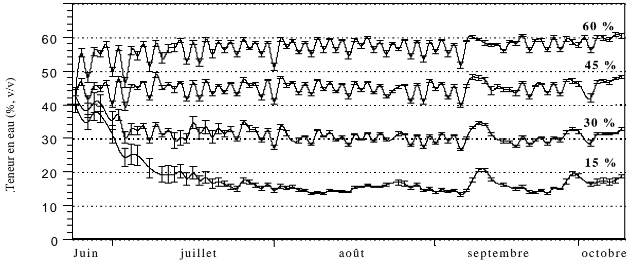
Figure 1. Exemple de contrôle très précis des quatre teneurs en eau (% v/v) dans le substrat, à l'aide de la RDT.
