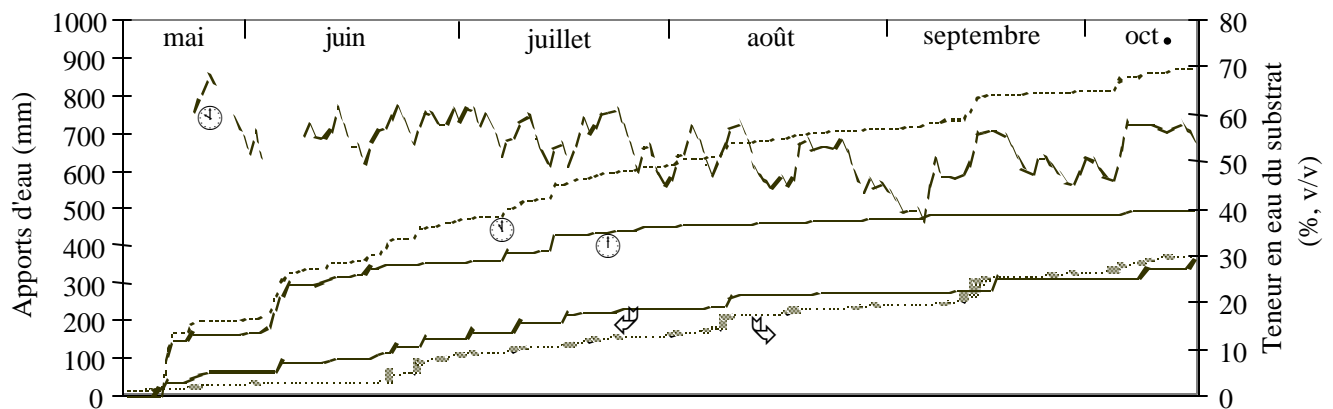
Figure 2. Évolution saisonnière : \circ teneurs en eau (% v/v) du substrat, \square apports d'eau cumulatifs, \triangle irrigations cumulatives, \triangleleft pertes d'eau cumulatives et \otimes pluies cumulatives.
